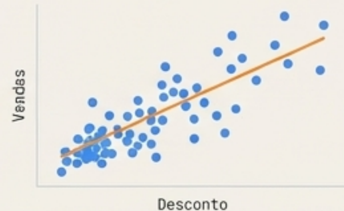
Gráfico de Dispersão (Scatter)
